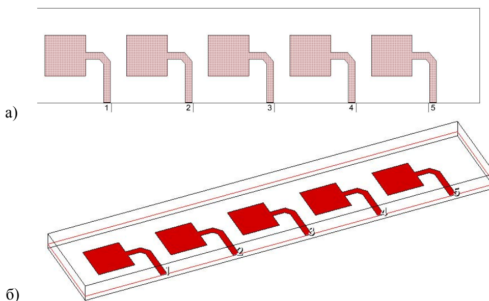
Рис. 1. Созданная топология излучающей части микрополосковой антенной решетки (а) и ее трехмерный вид (б)
