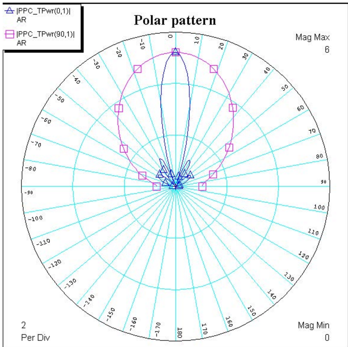
Рис. 2. Диаграмма направленности микрополосковой антенной решетки в двух взаимно ортогональных плоскостях
